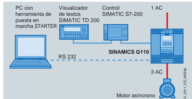
Ejemplo de configuración de SINAMICS G110 (variante USS con SIMATIC S7-200, conexión PC-convertidor con juego opcional para conexión a PC)
