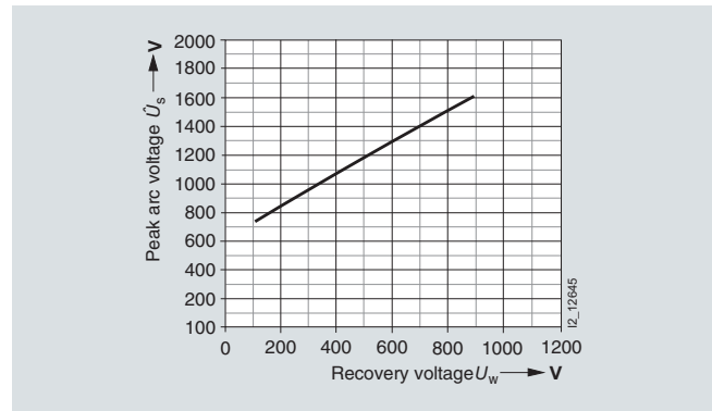
Example: 3NE4 333-0B SITOR fuse link
