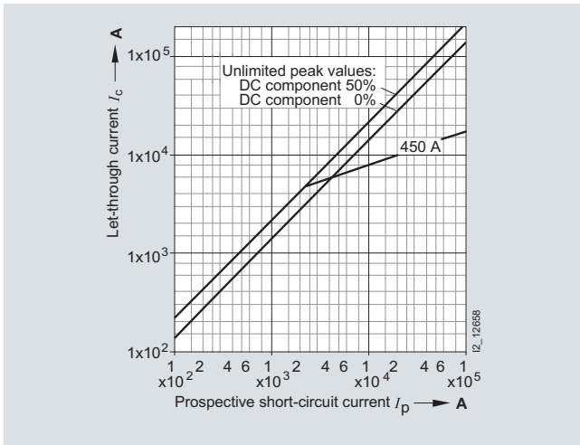
Example: 3NE4 333-0B SITOR fuse link
