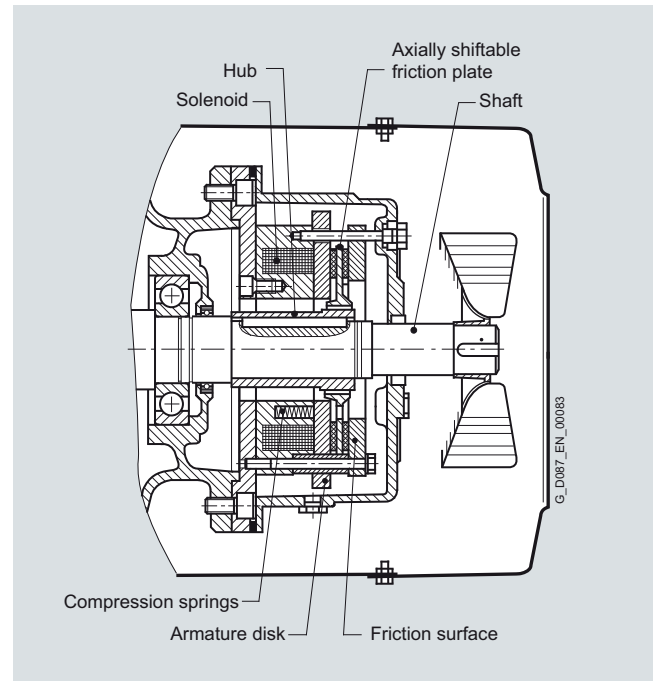
KFB brake
