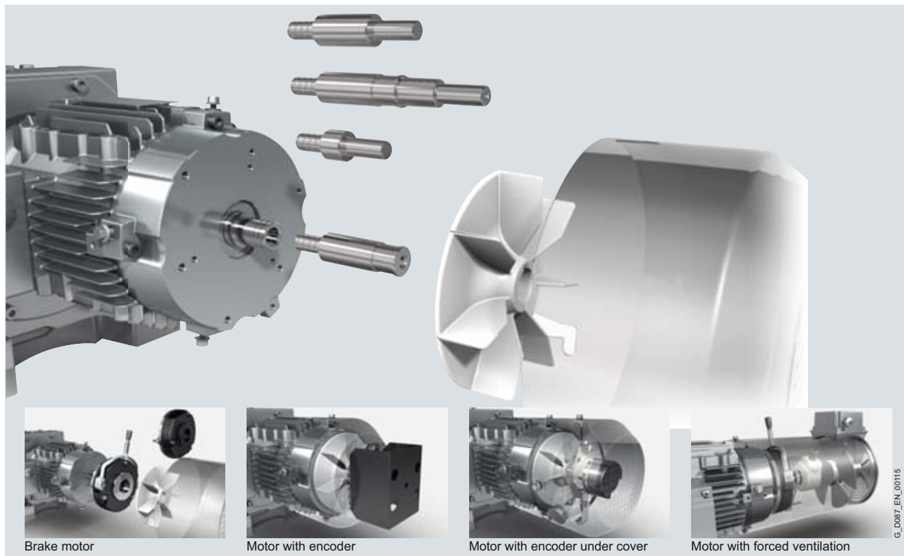
Brake motor
